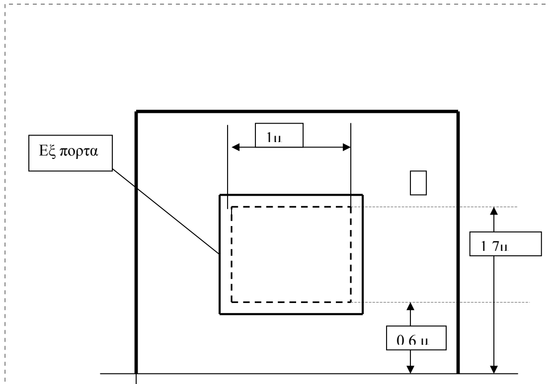
Τυπική όψη ορόφου πλευράς Γ
