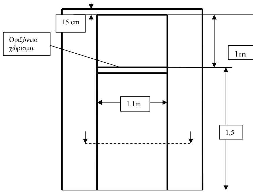
ΑΝΟΙΓΜΑΤΑ ΚΑΜΠΙΝΑΣ
