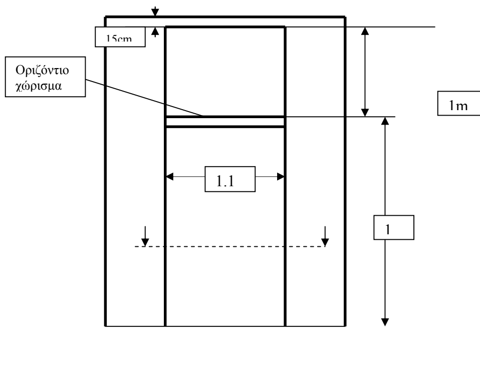
ΑΝΟΙΓΜΑΤΑ ΚΑΜΠΙΝΑΣ
