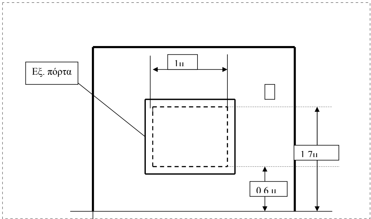
Τυπική όψη ορόφου πλευράς Γ
